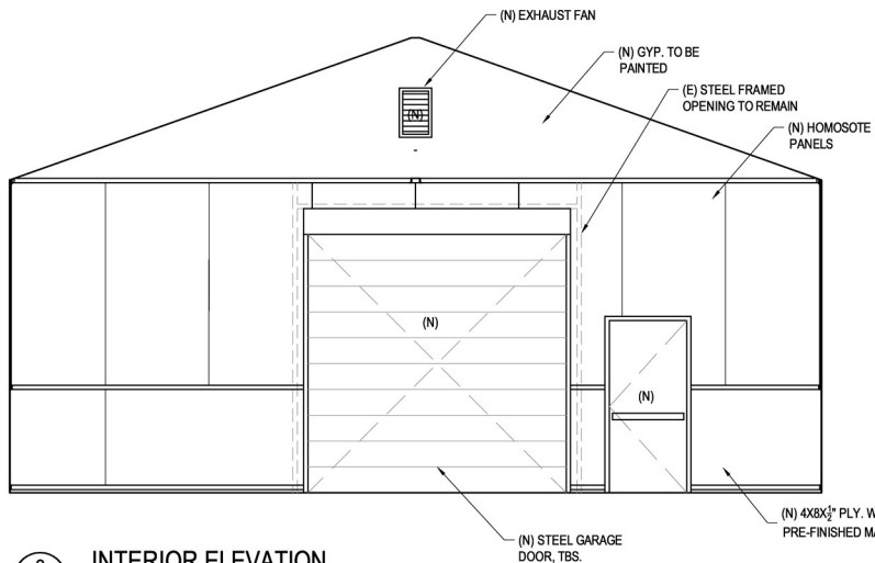
2 A3 INTERIOR ELEVATION SCALE: 1/4" = 1'
