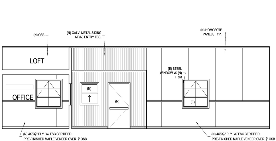
1 A3 INTERIOR ELEVATION SCALE: 1/4" = 1'
